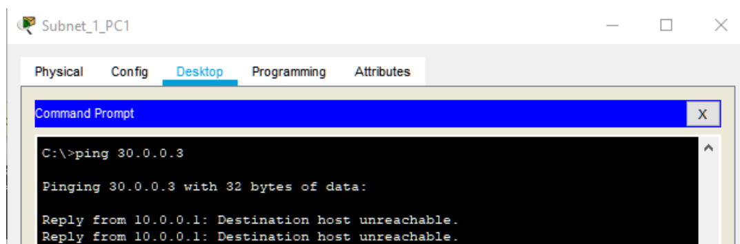
Εικόνα 6.7: Ανεπιτυχής δοκιμή λειτουργίας επιπέδου δικτύου προς έναν Η/Υ που ανήκει σε άλλο υποδίκτυο
