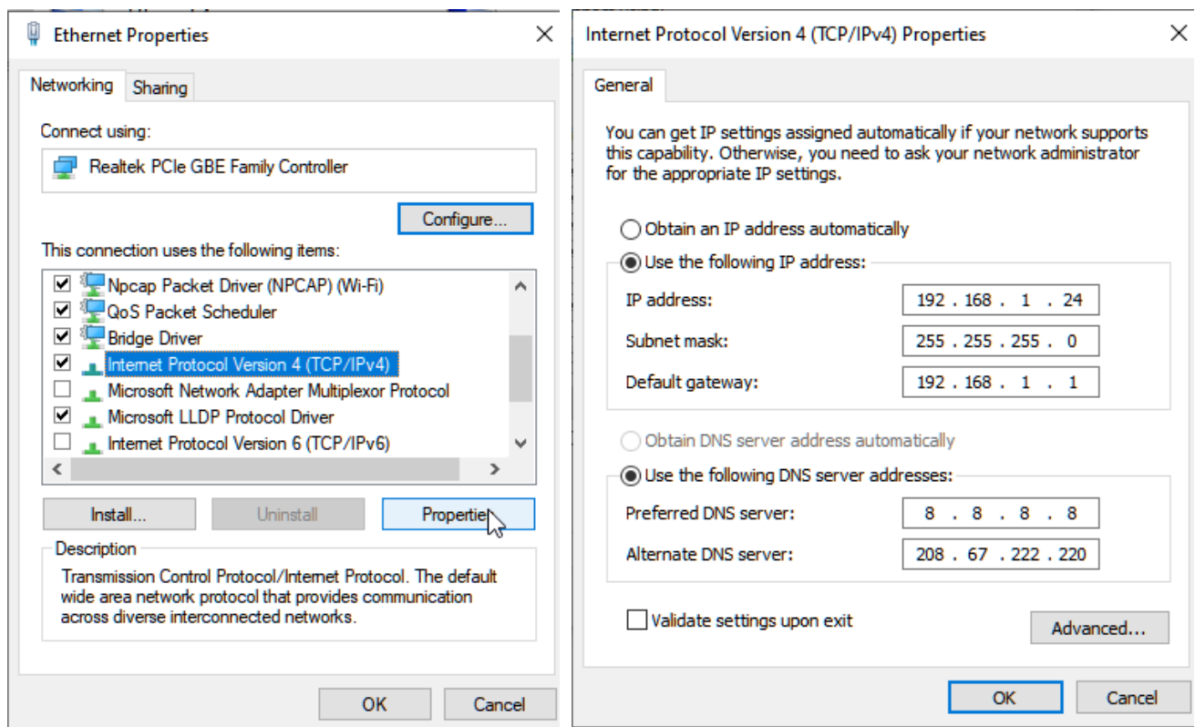
Εικόνα 6.3: Ρυθμίσεις των πρωτοκόλλων επιπέδου δικτύου σε λειτουργικό σύστημα Windows 7/8.1/10: Αριστερά: Επιλογή του IPv4 ως ενεργό πρωτόκολλο επιπέδου δικτύου με απενεργοποίηση του IPv6. Δεξιά: Ανάθεση ζεύγους IP address, Subnet mask. Επίσης ανάθεση Default Gateway και DNS servers της Google (8.8.8.8) και της OpenDNS (208.67.222.220)
