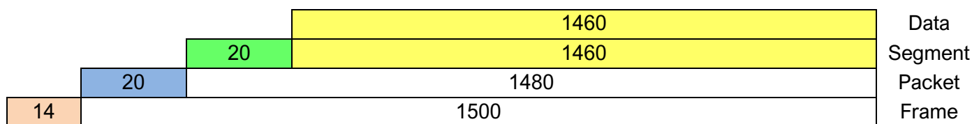
Εικόνα 4.6: Μέγιστος αριθμός Bytes σε κάθε επίπεδο με TCP στο L4.
