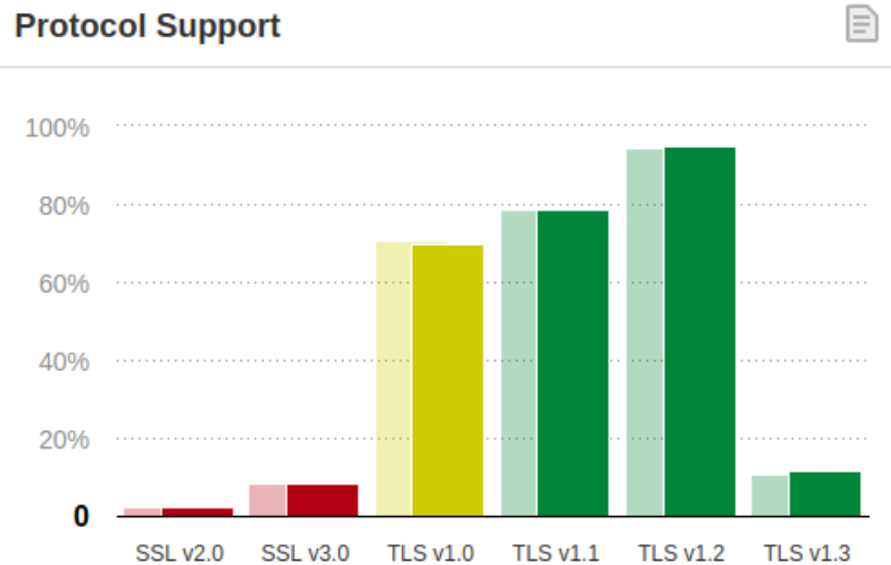
Εικόνα 4.9: Οι διαφορετικές εκδόσεις TLS που χρησιμοποιούνται σήμερα (Φεβρουάριος 2019). Πηγή: https://medium.com/iocscan/transport-layer-security-tls-ssl-8e02b6d1d648
