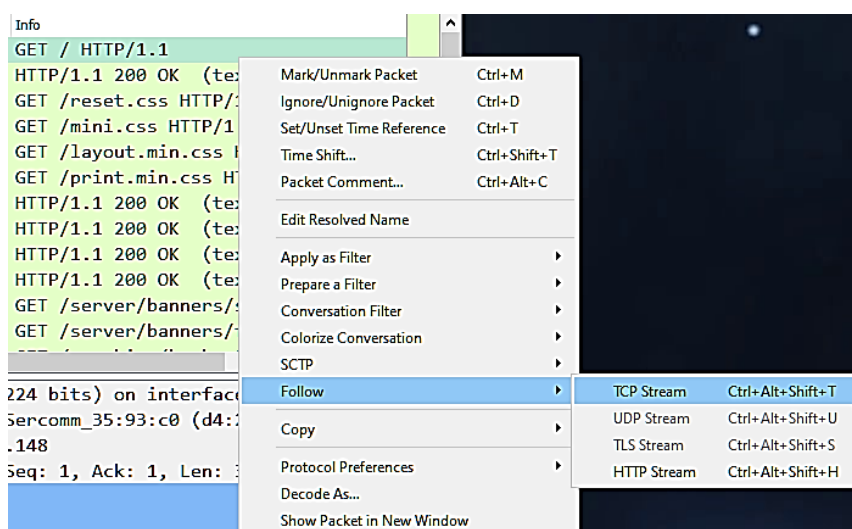
Εικόνα 4.8: Λειτουργία FollowTCPStream από γραμμή αιτήματος HTTP.
