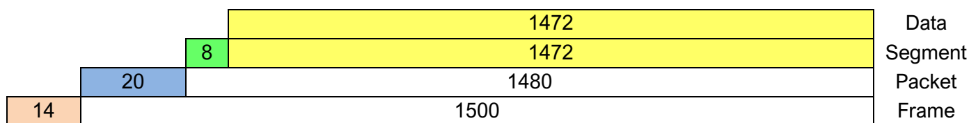
Εικόνα 3.18: Μέγιστος αριθμός Bytes σε κάθε επίπεδο με UDP στο L4.
