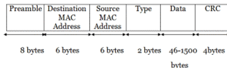
Εικόνα 3.14: Bytes σε κάθε πεδίο για πλαίσιο Ethernet.
