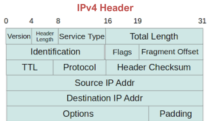
Εικόνα 3.15: Bytes σε κάθε πεδίο για πακέτο IPv4, με κάθε γραμμή να αντιστοιχεί σε 32 bytes.
