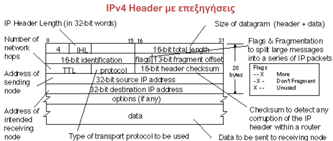
Εικόνα 3.16: Bytes σε κάθε πεδίο για πακέτο IPv4, με επεξηγήσεις.
