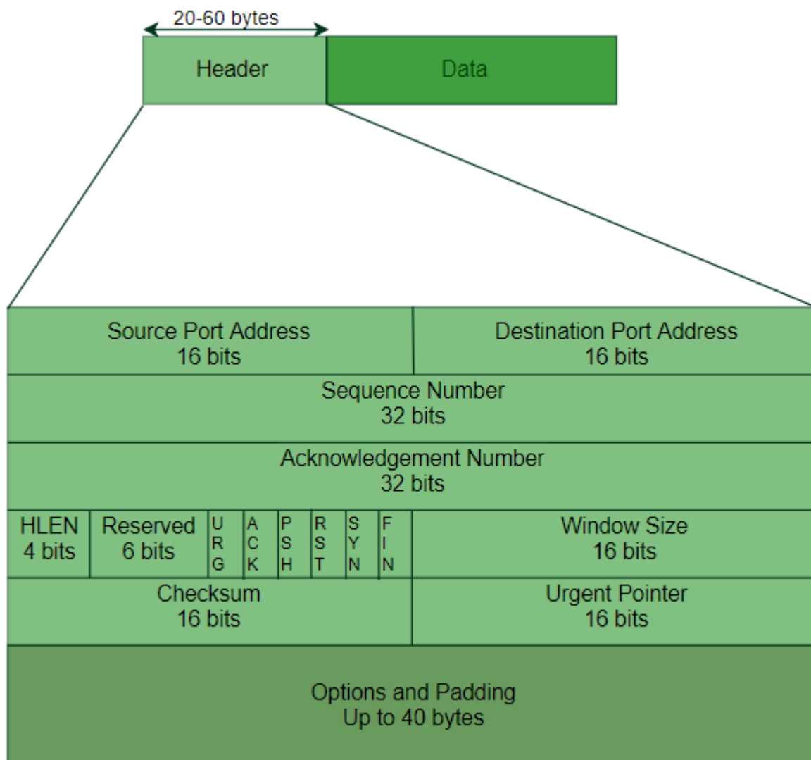
Εικόνα 4.7: TCP header.
