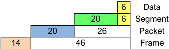
Εικόνα 4.5: Ελάχιστος αριθμός Bytes σε κάθε επίπεδο με TCP στο L4.
